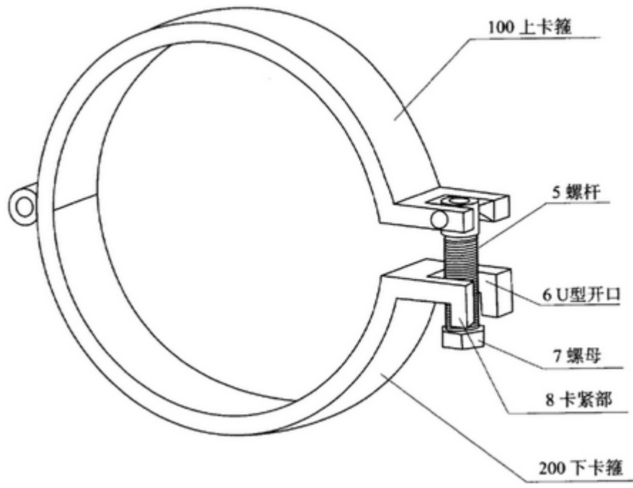
图 6 第三实施例示意图
