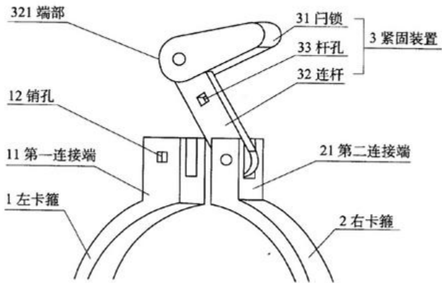
图 1 第一实施例打开状态示意图
