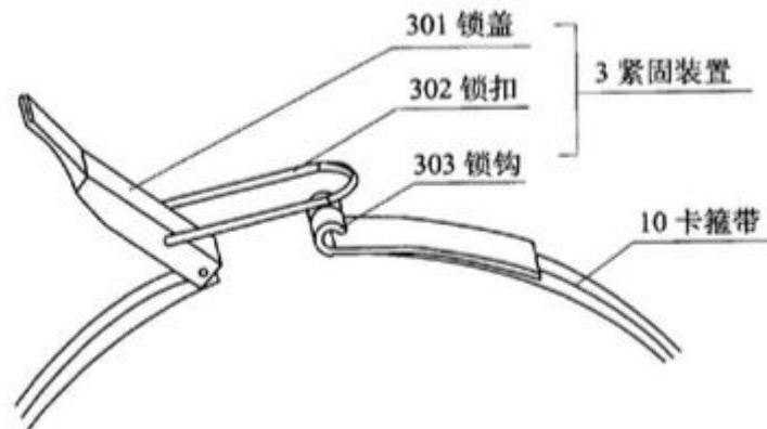
图 5 第二实施例打开状态示意图
