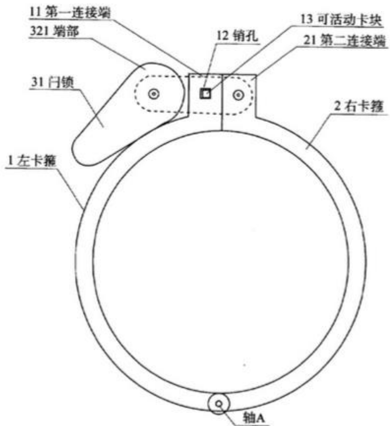
图 2 第一实施例锁紧状态示意图
