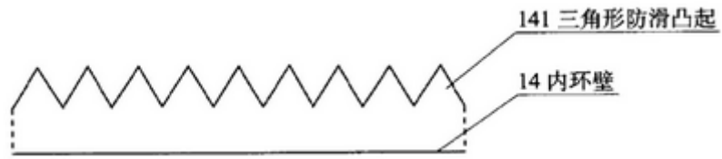
图 3 第一实施例橡胶垫圈局部放大图
