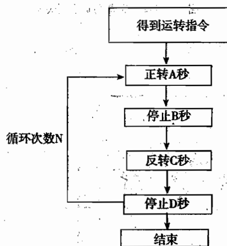
图 4 电路控制器件循环正反转控制步骤图
