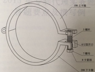
图 6 第三实施例示意图
