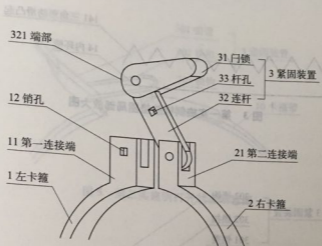
图 1 第一实施例打开状态示意图
