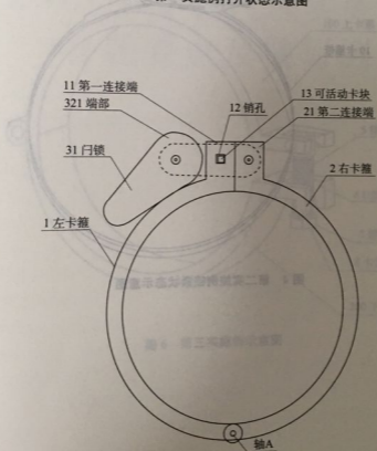
图 2 第一实施例锁紧状态示意图
