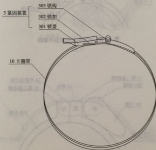
图4 第二实施例锁紧状态示意图
