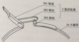
图 5 第二实施例打开状态示意图
